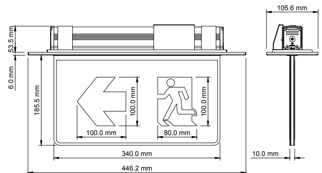
Dimensions
